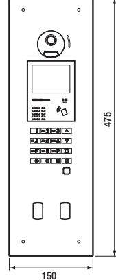
Encastrement 446 x 125 x 60 mm
