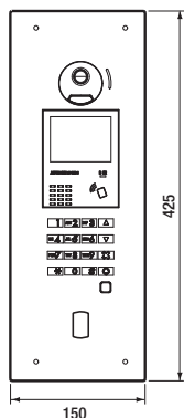
Encastrement avec GT4B
