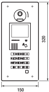
Encastrement avec GF3B
