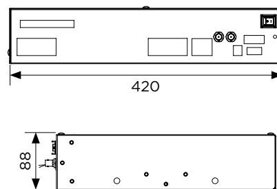
Dimensions : 2U, 19"
